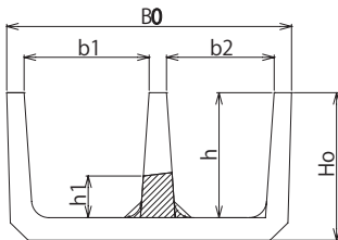
正面図 鉄筋コンクリートU形タイプ
