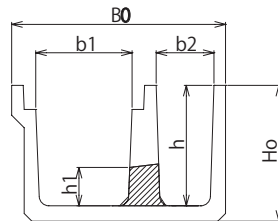
正面図 CH25タイプ 道路用鉄筋コンクリート側溝タイプ
