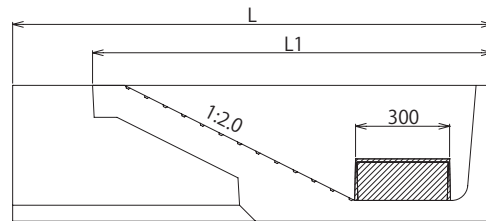
側断面図
